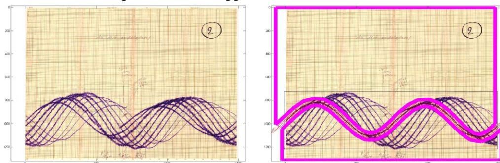
Figure 3 : Exemple d'utilisation de polygone supprimant les éléments à une certaine distance de la marée prédite (marégramme de Port-Tudy fourni par le SHOM)
