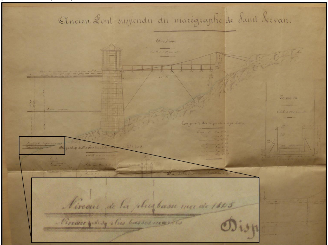
Figure 6 : Plan du marégraphe de Saint-Servan avec un zoom sur le niveau de référence de l'époque (source : SHD Vincennes - DD_2_2576 Chemise Marégraphe Saint-Servan)
