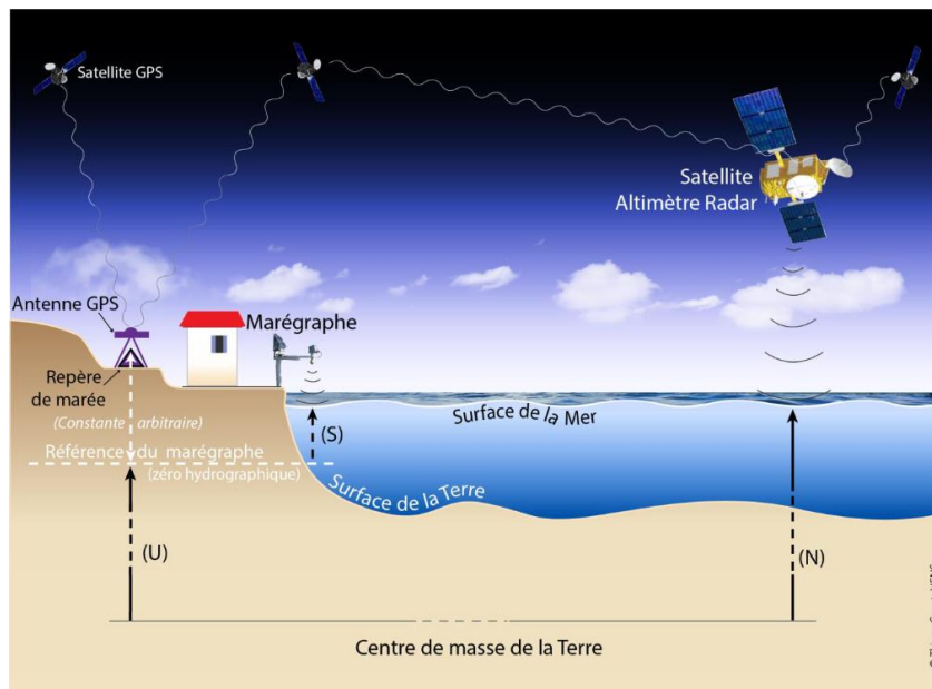
Figure 5 - Description schématique d'une station marégraphe co-localisée avec un récepteur GNSS pour la détermination de la hauteur ellipsoïdale du niveau de la mer et pour la mesure des mouvements verticaux du sol. La mesure du niveau de la mer par l'altimétrie par rapport au géoïde* est également représentée (crédits : Thierry Guyot, LIENSs).
