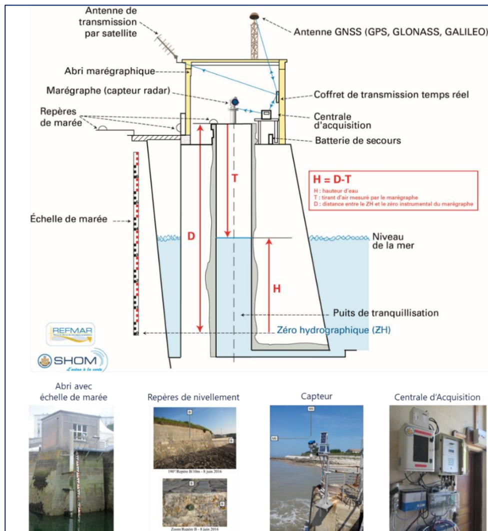
Figure 4 - Exemple d'un observatoire de marée idéal.
