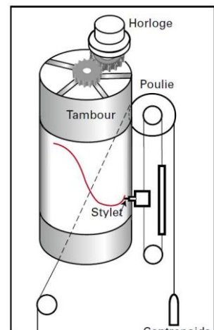
Figure 2 - Principe du marégraphe à flotteur (source : Shom)
