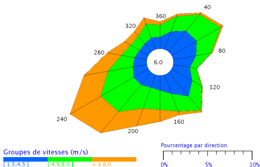
Figure 5 - Exemple de rose des vents établie à partir des observations au sémaphore de Boulogne-sur-Mer (sur la période 1981-2010) (Source : Météo-France). Les vents prédominants viennent du secteur sud-ouest (entre le 220 et le 260), notamment pour les vents forts (> 8m/s) et modérés (4,5 à 8 m/s) ; le secteur nord-est (entre 140 et 180°) arrive ensuite, notamment pour les vents plus faibles (entre 1,5 et 4,5 m/s).
